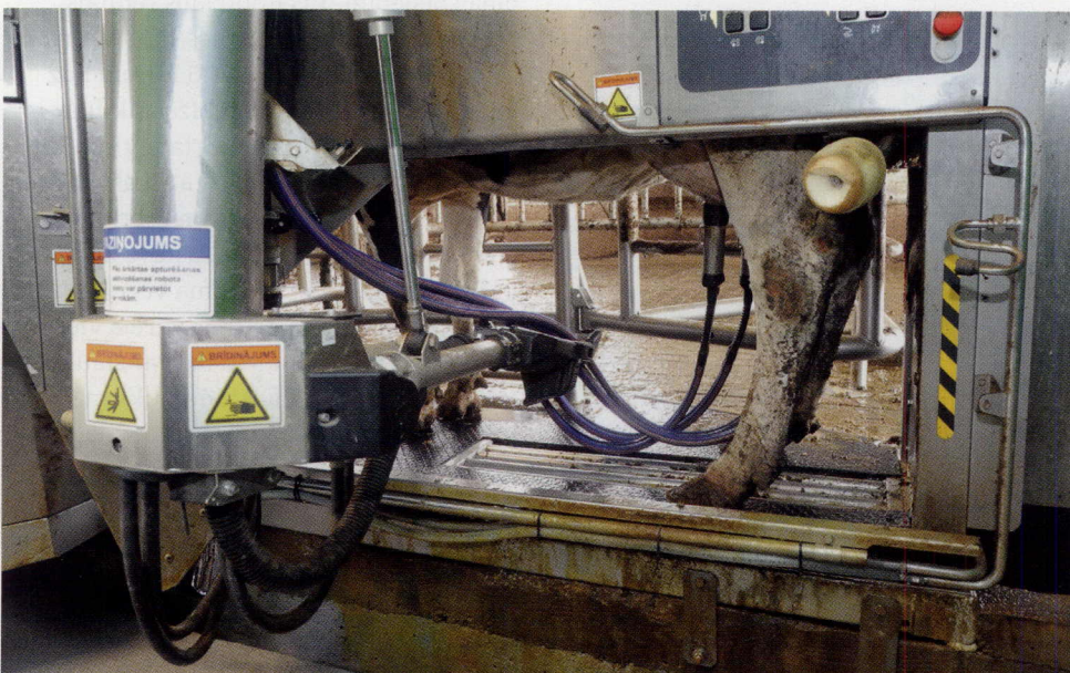
"De Laval" slaukšanas robots darbībā. Saimniecība šo zīmolu izvēlējās pēc agrākās sadarbības izvērtējuma un pakalpojumu centra atrašanās vietas.
